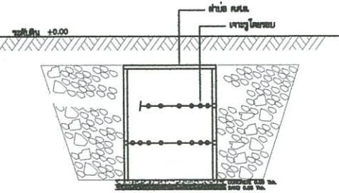
แบบขยายบ่อซึม
