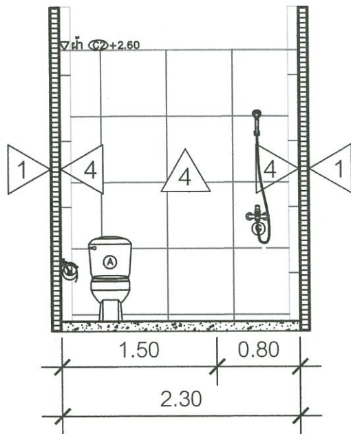
แบบขยาย ห้องน้ำ รูปตัด A
