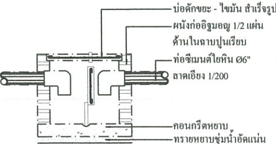
แบบขยายบ่อพักขยะ - ไขมัน(MH - 2)
