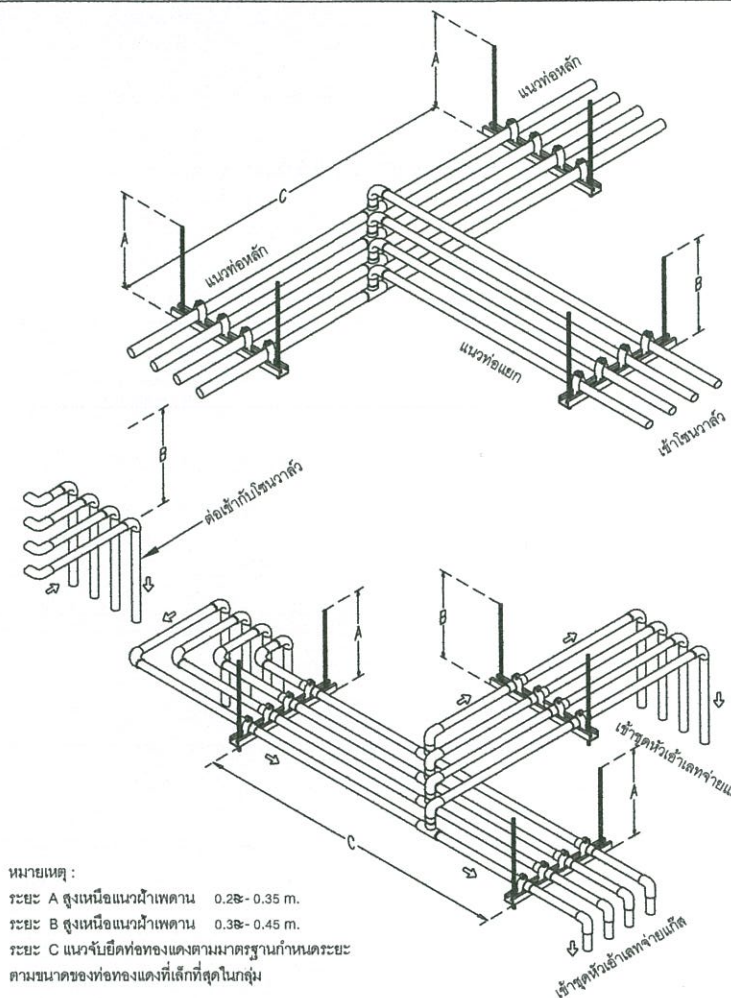
รูปขยายแนวการเดินท่อจ่ายแก๊ส
