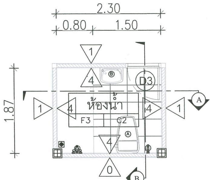
แบบขยาย ห้องน้ำ
