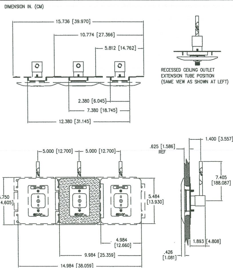
DETAIL "A" (WALL OUTLET GAS)
